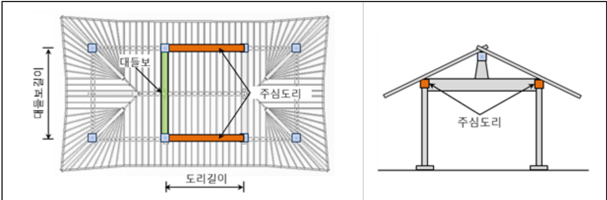
그림 4.5-1 3량가구 형식의 지붕도리의 구성 및 관련 용어
