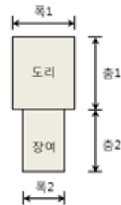
(b) 방형단면-방형단면의 등가 겹침부재
