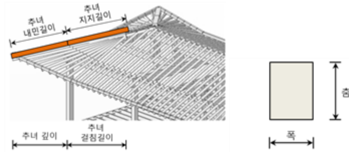
단면의 정의
