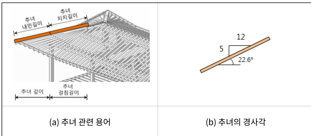
그림 4.2-1 추녀 관련 용어 및 추녀의 경사각
