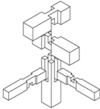
(d) 우주에 장여,도리가 접합된 접합부
