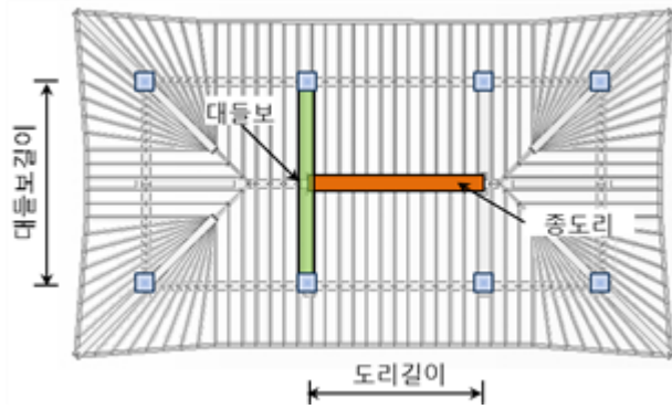
(b) 3량가구 형식의 종도리 및 관련 용어
