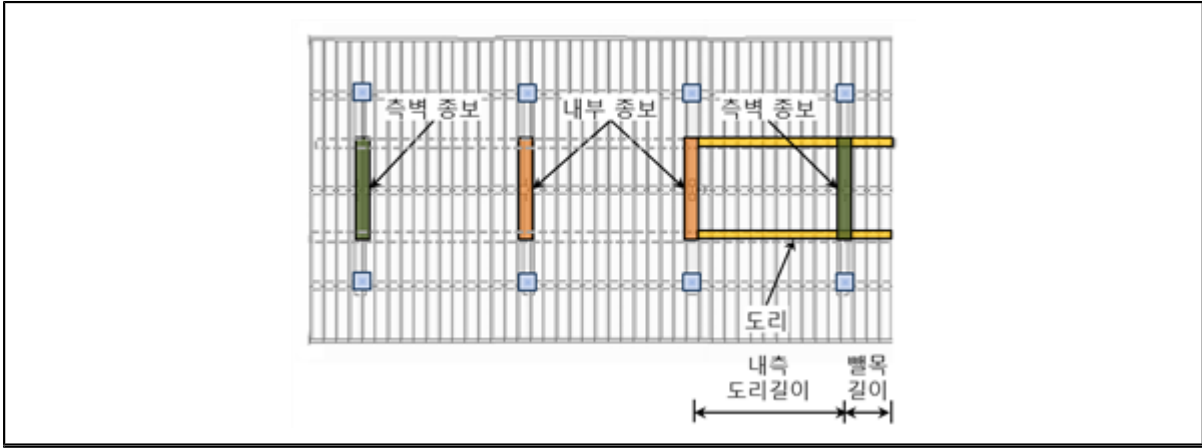
그림 4.4-2 맞배지붕의 측벽 종보
