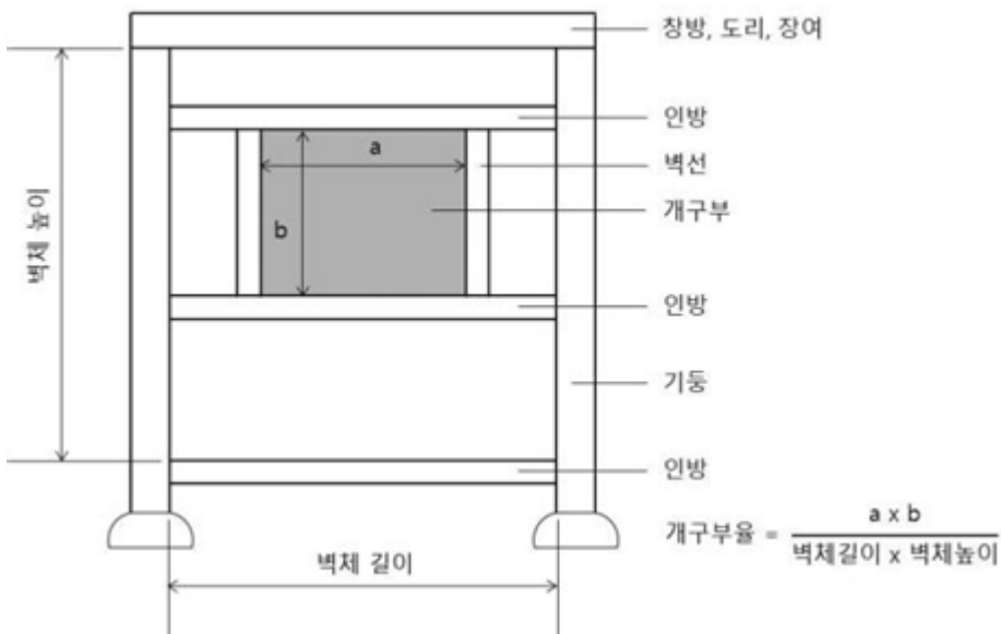
그림 4.10-5 벽체길이, 높이와 개구부율
