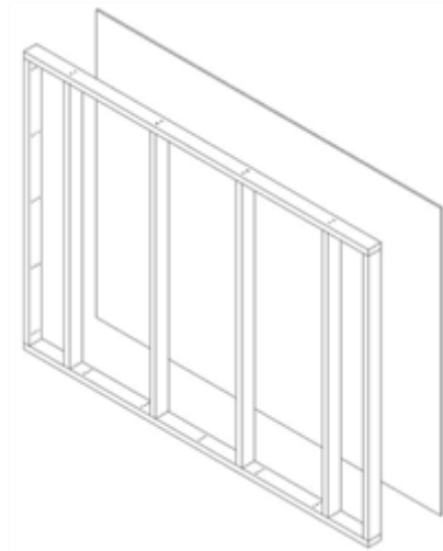
그림 4.10-2 판재중깃 한쪽에 배치된 구조용목질판재
