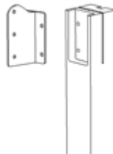
(e) 3개의 연결볼트를 이용한 기둥과 대들보의 철물접합
