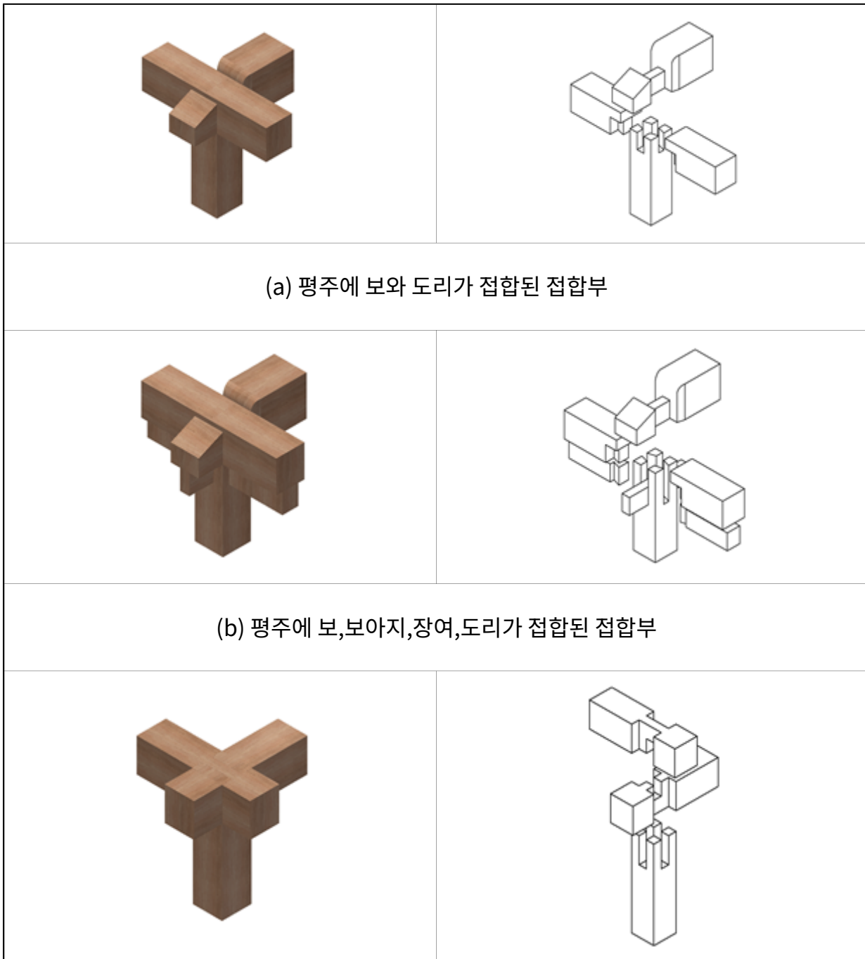
그림 4.9-2 전통접합부 예시
