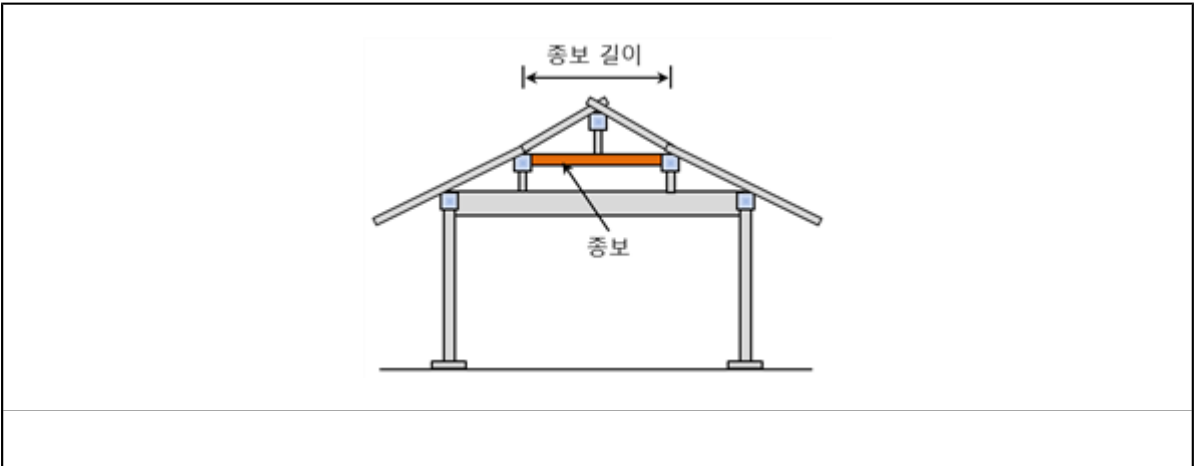
그림 4.4-1 종보의 구성 및 관련 용어
