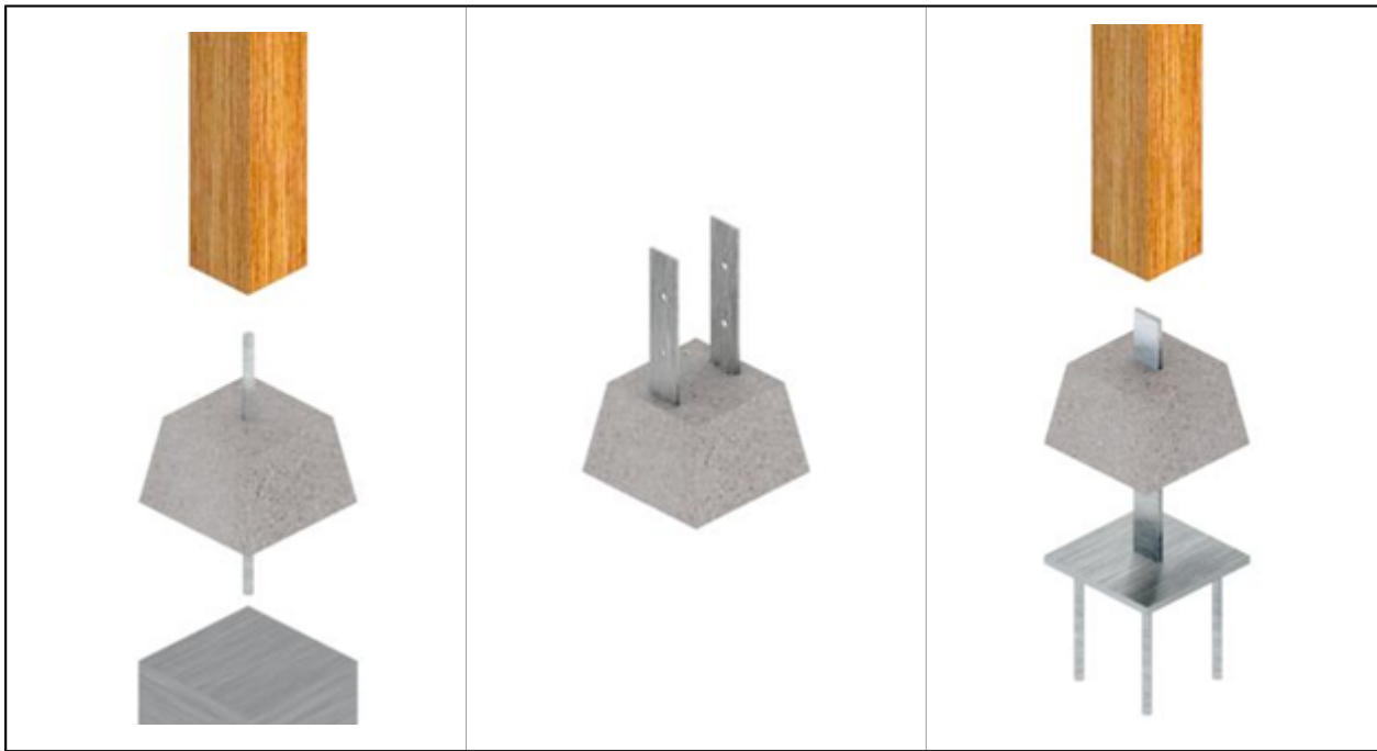
그림 4.9-2 전통접합부 예시
