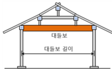
(b) 5량가구 형식의 대들보
