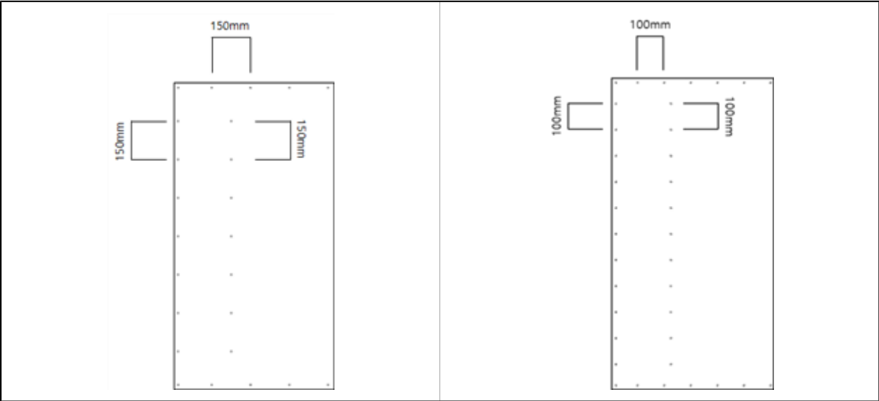
그림 4.10-4 못박기 간격 예시(150mm, 100mm)
