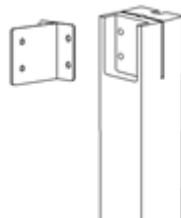
(c) 2개의 연결볼트와 받침재를 이용한 기둥과 도리의 철물접합
