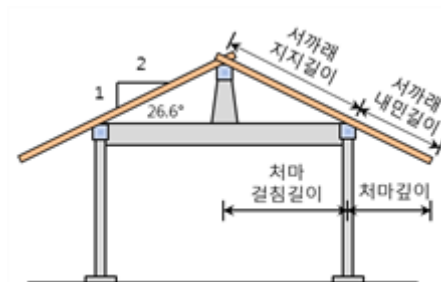
3량가 서까래
