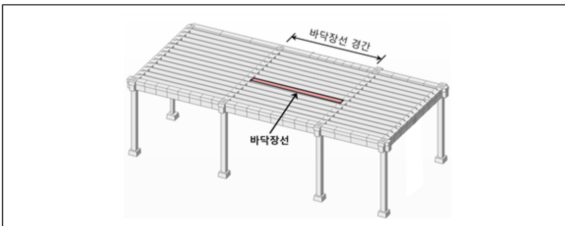
그림 4.7-1 바닥장선의 구성 및 관련 용어
