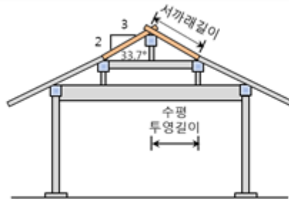
5량가 단면
