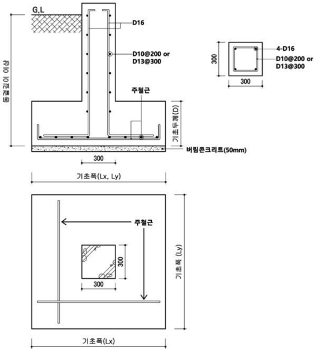
그림 4.11-3 독립기초 (단위: mm)
