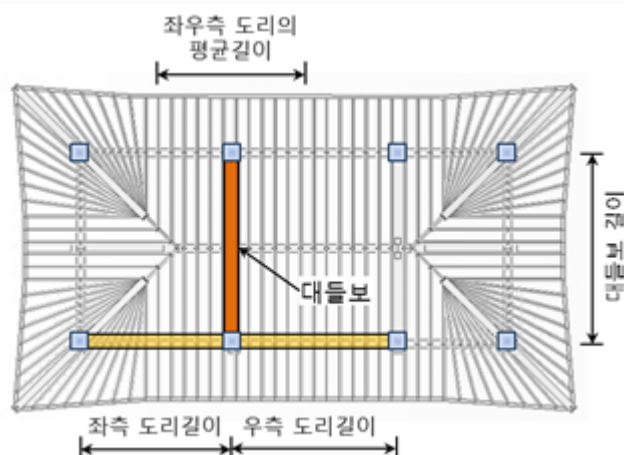
(a) 3량가구 형식의 대들보
