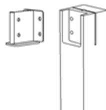
(c) 2개의 연결볼트와 받침재를 이용한 기둥과 도리의 철물접합
